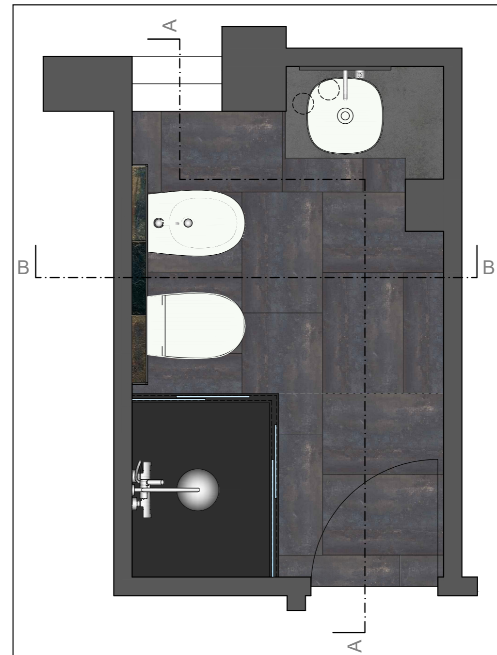
PLANIMETRIA BAGNO
