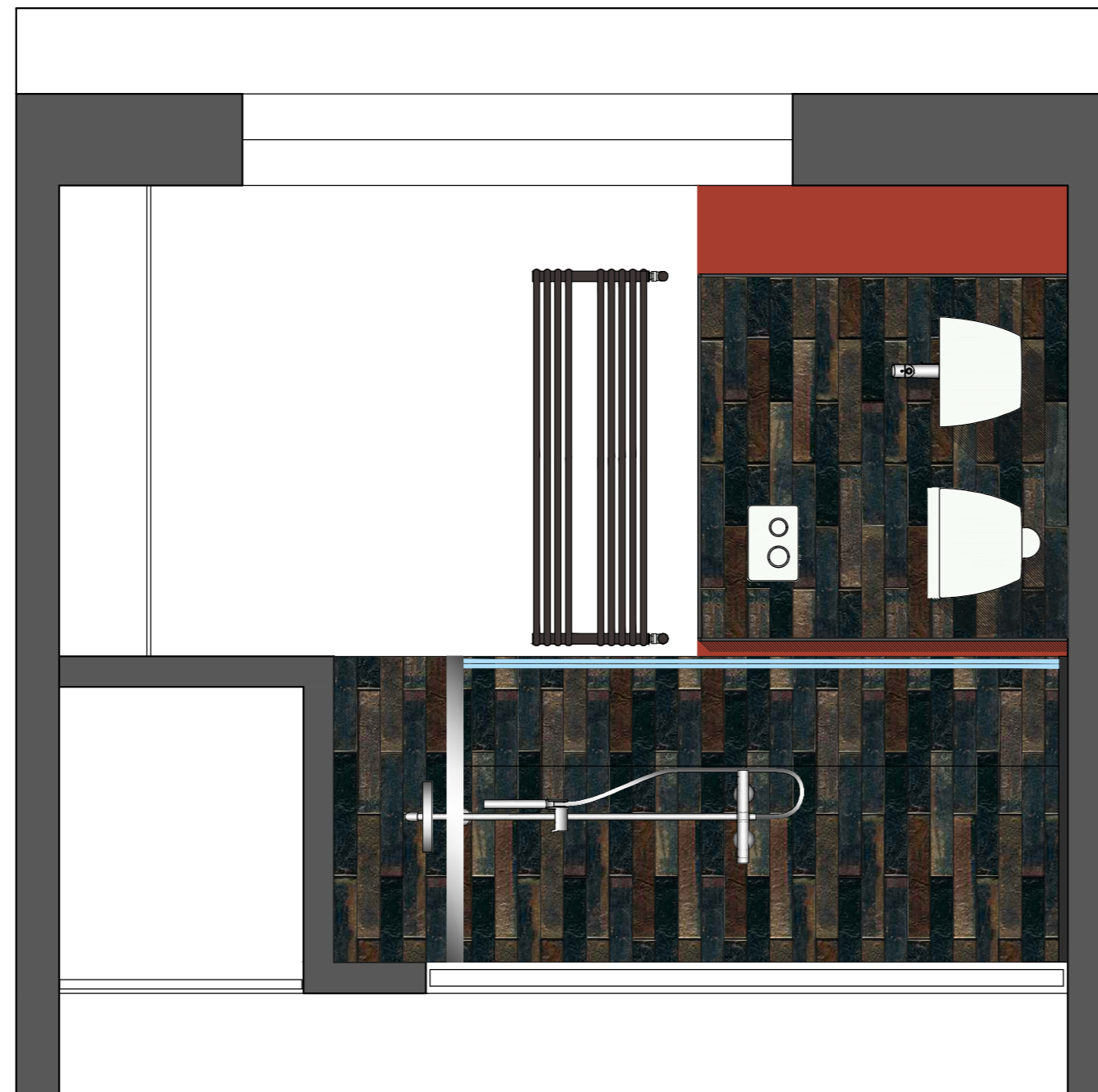
SEZIONE A-A
