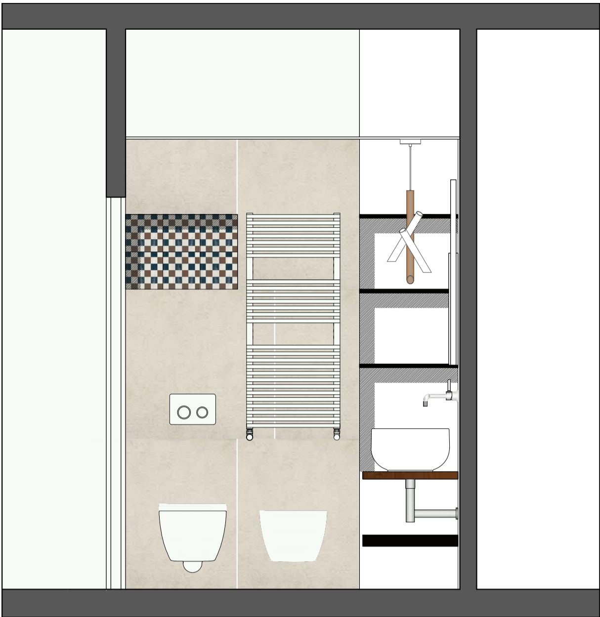
SEZIONE A-A
